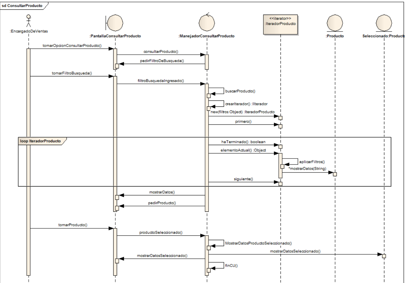
Diagrama de secuencia Consultar Producto- Patrón Iterator
