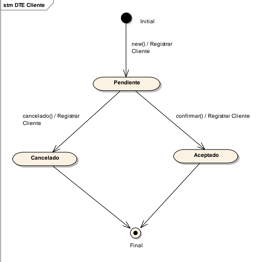
Diagrama de estados Cliente
