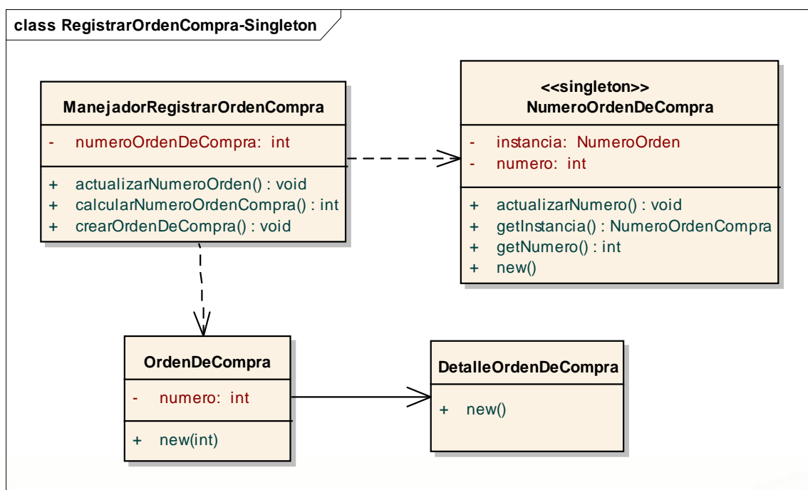
Diagrama de diseño Registrar Orden de Compra
