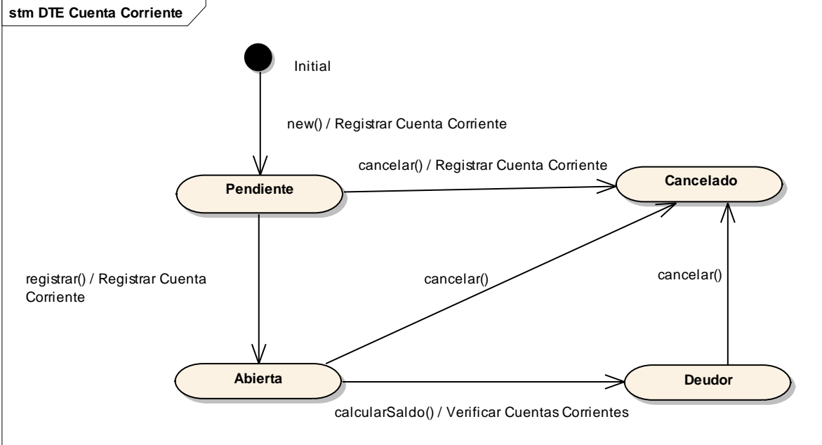
Diagrama de estados de la clase Cuenta Corriente
